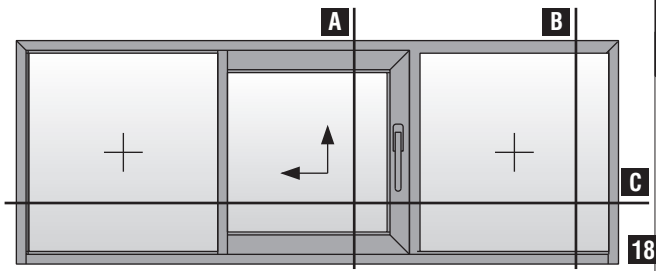
Μονόφυλλο ανασυρόμενο με σταθερά One sash lift & slide with fixed
