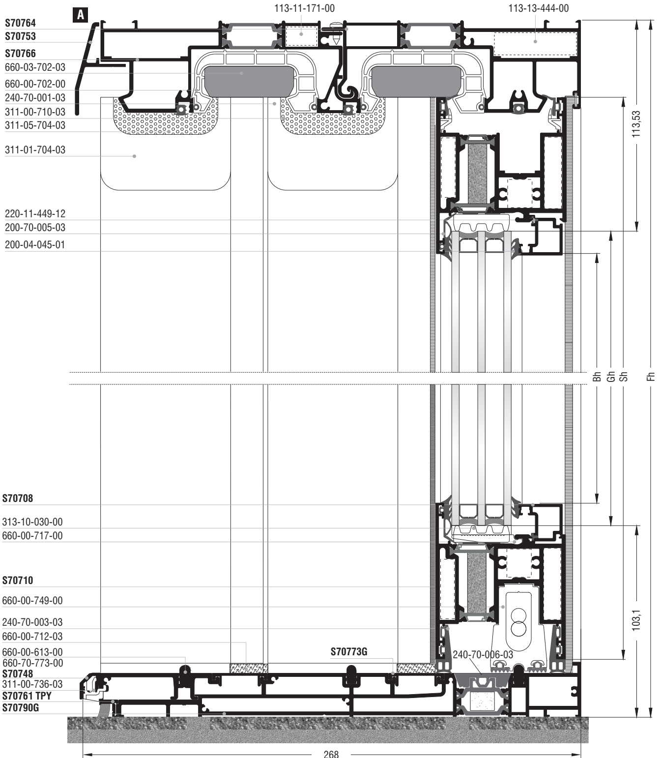
Εξάφυλλο επάλληλο φιλητό ανασυρόμενο με χρήση τριπλού οδηγού & χαμηλού οδηγού S70790G Six sash parallel meeting stile lift & slide with triple frame guide & S70790G short frame guide use
