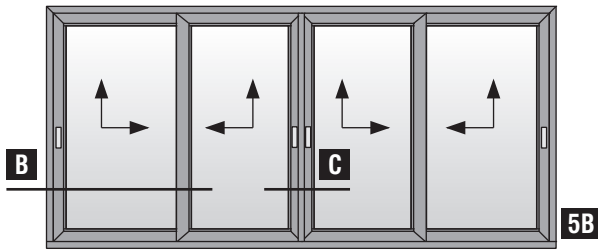
Τετράφυλλο φιλιτό επάλληλο ανασυρόμενο με χρήση χαμηλού οδηγού S70786 | Four sash parallel meeting stilet lift & slide with S70786 short frame guide use
