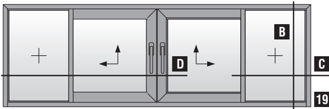
Δίφυλλο φιλητό αριστερά ανασυρόμενο με σταθερά Two sash meeting stile left lift & slide with fixed
