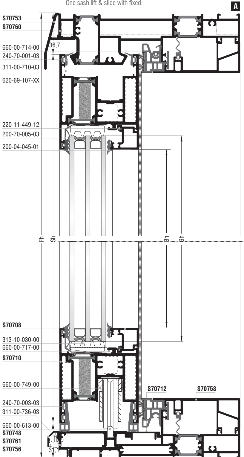
Μονόφυλλο ανασυρόμενο με σταθερά One sash lift & slide with fixed
