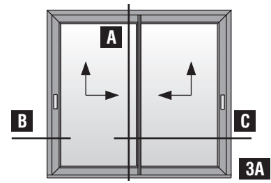
Δίφυλλο επάλληλο ανασυρόμενο ΔΕΞΙ με χρήση χαμηλού οδηγού S70786 (κοπή 90°) Two sash parallel lift & slide RIGHT with S70786 short frame guide use (90° cutting)
