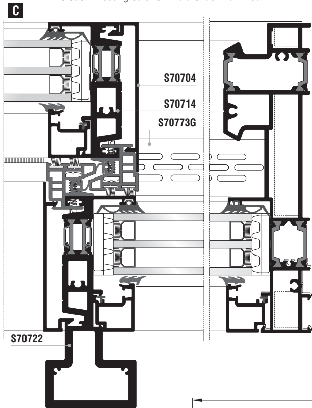
Δίφυλλο φιλητό αριστερά ανασυρόμενο με σταθερά Two sash meeting stile left lift & slide with fixed
