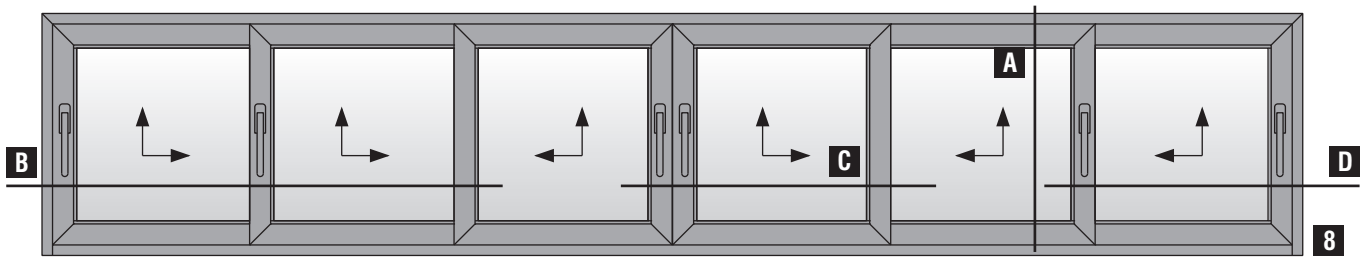
Εξάφυλλο επάλληλο φιλητό ανασυρόμενο με χρήση τριπλού οδηγού & χαμηλού οδηγού S70790G Six sash parallel meeting stile lift & slide with triple frame guide & S70790G short frame guide use
