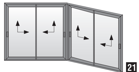
Τετράφυλλο επάλληλο (90° ΓΩΝΙΑ ΜΕΣΑ ) γωνιακής συνεργασίας κοπή 90° με χαμηλό οδηγό και χαμηλό φύλλο Four sash parallel slide (90° INTERIOR CORNER ) (90° cutting), with short frame guide use and short sash
