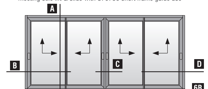
Τετράφυλλο φιλιτό επάλληλο ανασυρόμενο (κοπή 90°) με χρήση χαμηλού οδηγού S70786 Four sash meeting stile parallel lift & slide (90° cutting) with S70786 short frame guide use
