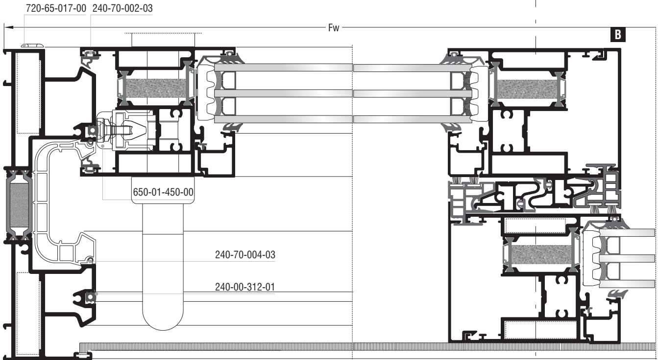
Τετράφυλλο φιλιτό επάλληλο ανασυρόμενο με χρήση χαμηλού οδηγού S70786 | Four sash parallel meeting stilet lift & slide with S70786 short frame guide use
