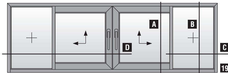
Δίφυλλο φιλητό αριστερά ανασυρόμενο με σταθερά | Two sash meeting stile left lift & slide with fixed
