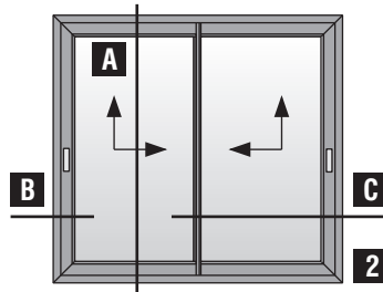
Δίφυλλο επάλληλο ανασυρόμενο παράθυρο (κοπή 90°) Two sash parallel lif & slide window (90° cutting)
