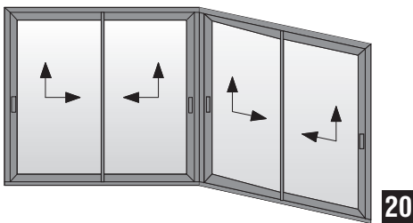
Τετράφυλλο επάλληλο (90° ΓΩΝΙΑ ΕΞΩ ) γωνιακής συνεργασίας κοπή 90° με χαμηλό οδηγό και χαμηλό φύλλο Four sash parallel slide (90° EXTERIOR CORNER ) (90° cutting), with short frame guide use and short sash
