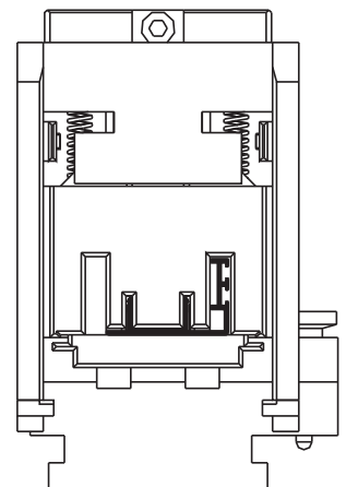
Αριστερή και δεξιά εισαγωγή Left and right insertion
