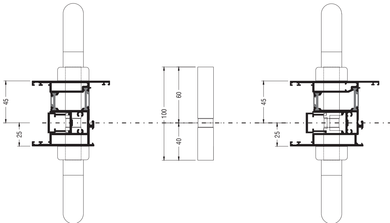
Κύλινδρος 40/60 - Cylinder 40/60
