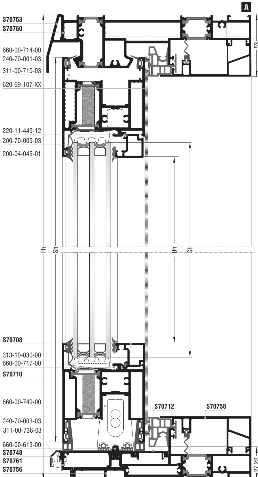
Δίφυλλο φιλητό αριστερά ανασυρόμενο με σταθερά Two sash meeting stile left lift & slide with fixed
