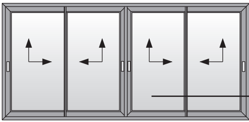
Τετράφυλλο φιλιτό επάλληλο ανασυρόμενο (κοπή 90°) Four sash meeting stile parallel lift & slide (90° cutting)
