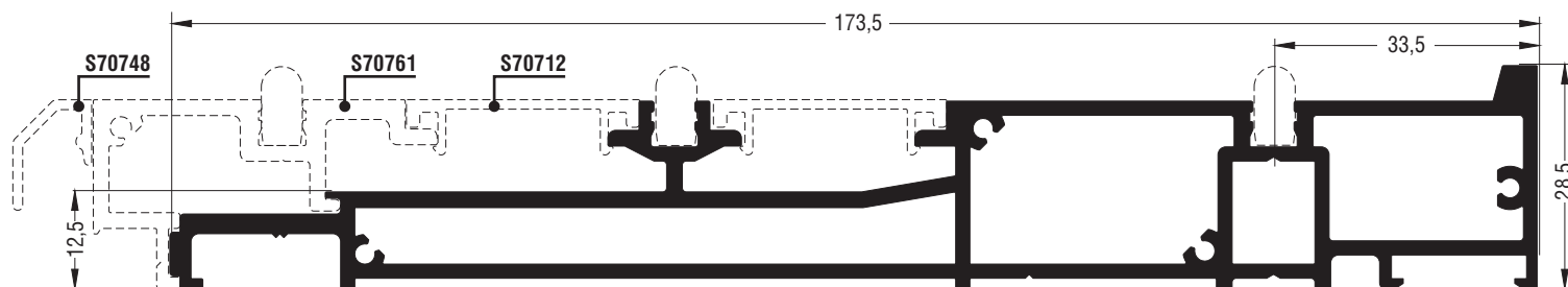
Προφίλ 1:2 | Profile 1:2
