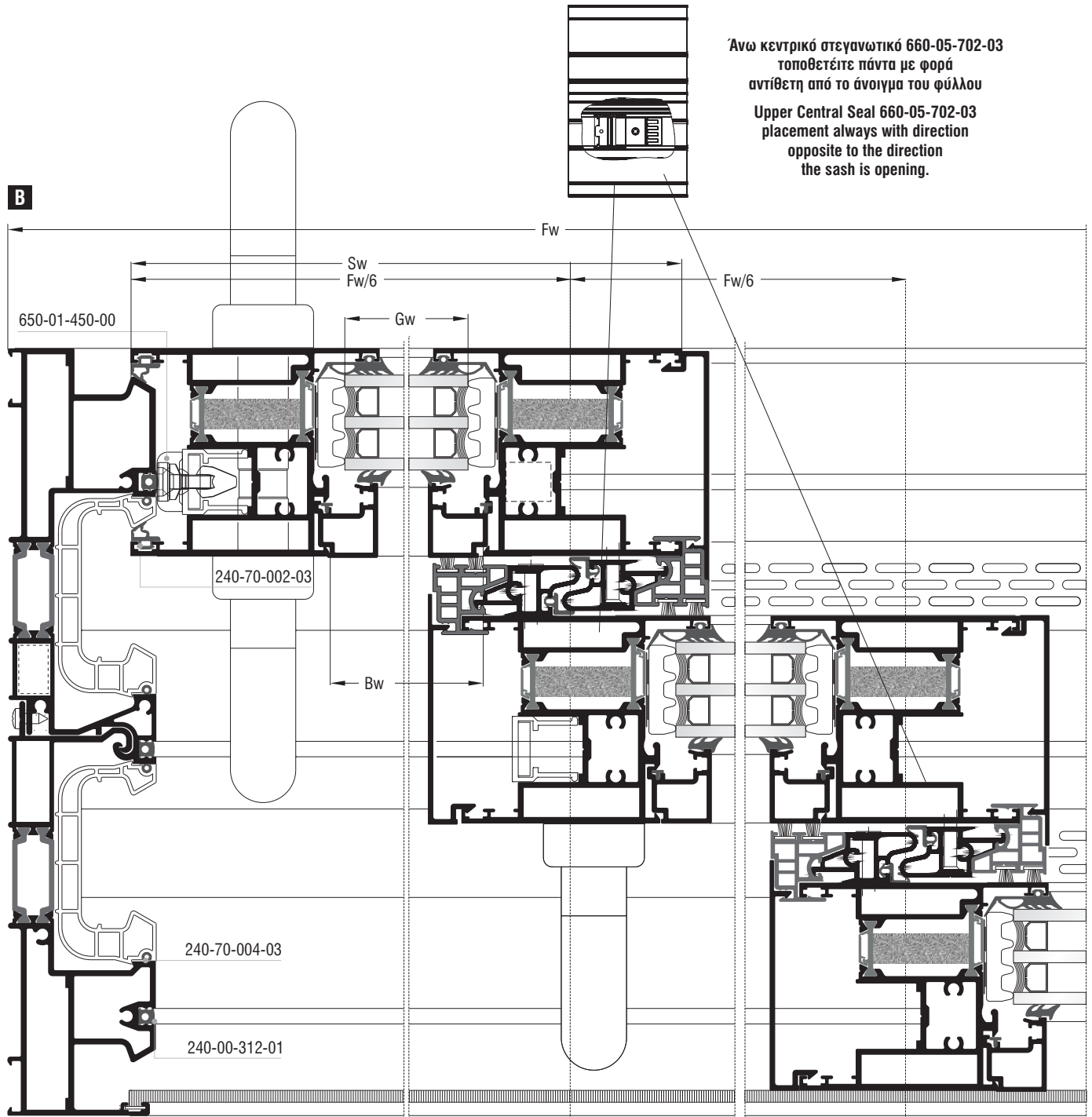
Εξάφυλλο επάλληλο φιλητό ανασυρόμενο με χρήση τριπλού οδηγού & χαμηλού οδηγού S70790G Six sash parallel meeting stile lift & slide with triple frame guide & S70790G short frame guide use
