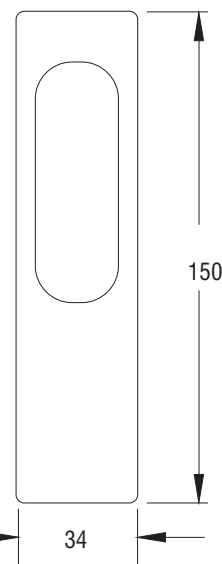
Εξωτερική χούφτα - External flush handle
