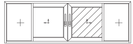
*Πρώτο φύλλο δεξί | Right sash first
