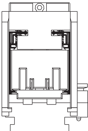
Αριστερή και δεξιά εισαγωγή Left and right insertion
