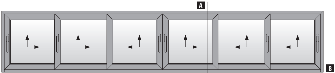
Εξάφυλλο επάλληλο φιλητό ανασυρόμενο με χρήση τριπλού οδηγού & χαμηλού οδηγού S70790G Six sash parallel meeting stile lift & slide with triple frame guide & S70790G short frame guide use
